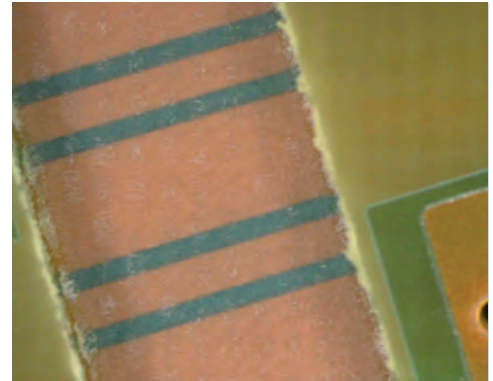
Fig. 62: Deep milling
