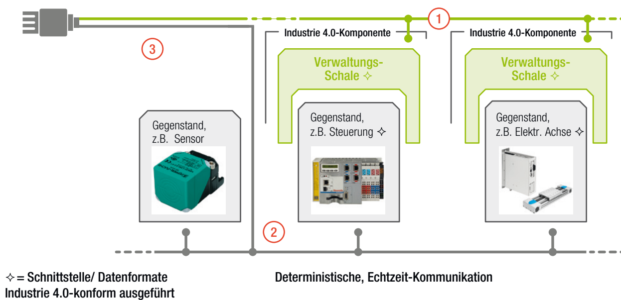
Abbildung 26: Kapselfähigkeit und Vernetzung einer Industrie 4.0 Komponente
