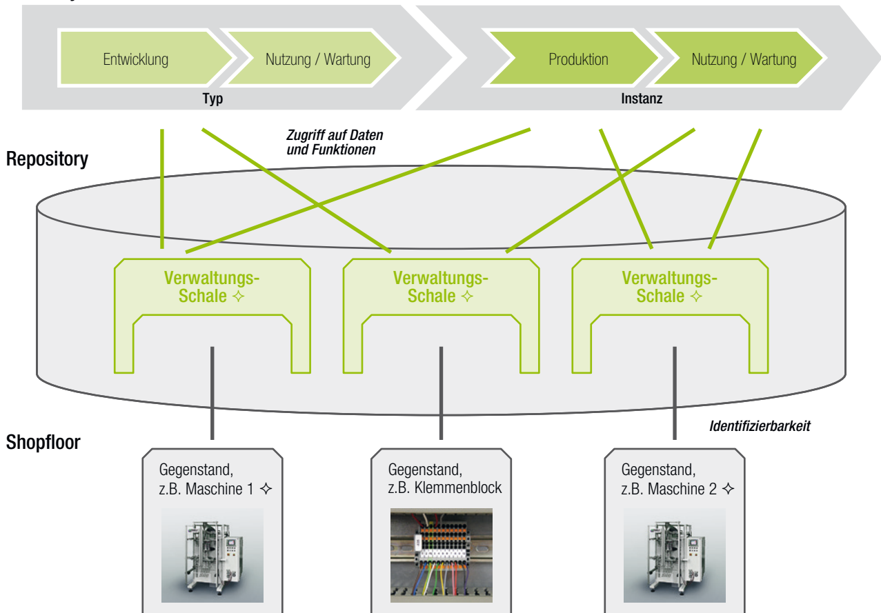
Abbildung 24: Repository
