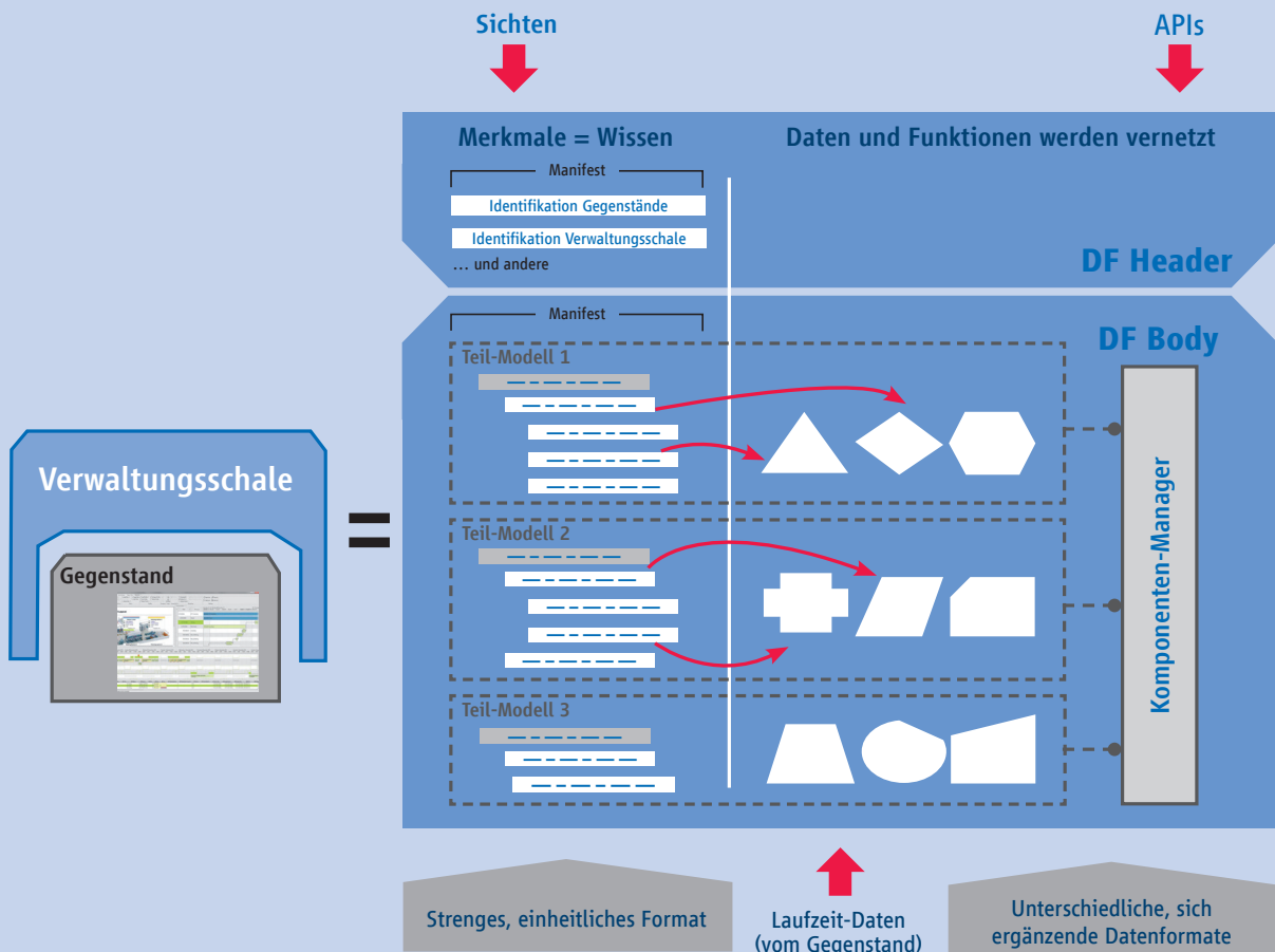
Abb. 4: Mögliche Header-/Body-Struktur
