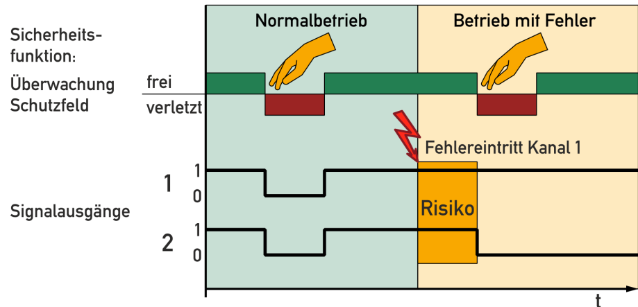
Abb. 1: Betrachtung eines redundanten Systems gemäß ISO 13849-1
