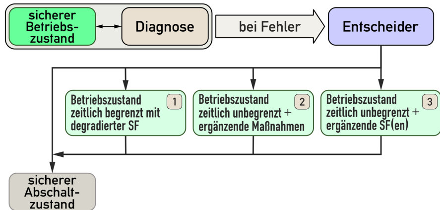
Abb. 10: Zustandsübergänge
