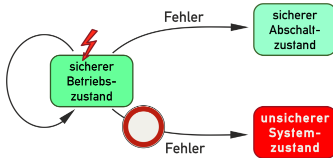
Abb. 4: System mit sicherer Überwachungsfunktion
