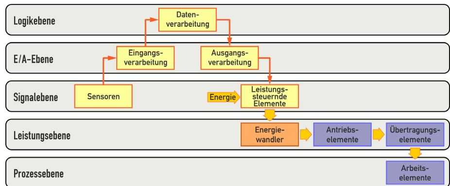
Abb. 3: Schematische Darstellung einer Maschinensteuerung
