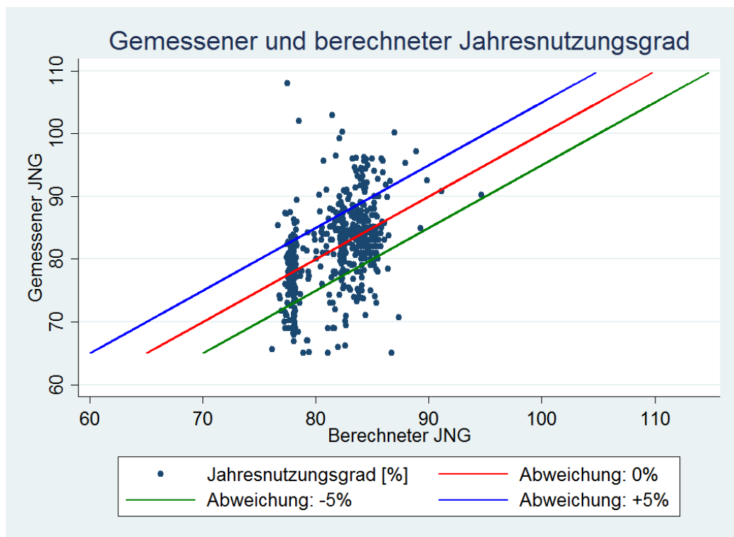
Abbildung 10: Zielkorridor und Fehleranalyse gemessener und berechneter Werte ( \pm 5\% Intervall)
